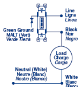
STRIP GAGE GABARIT DÉNUDAGE MEDIDA DE PELADO
